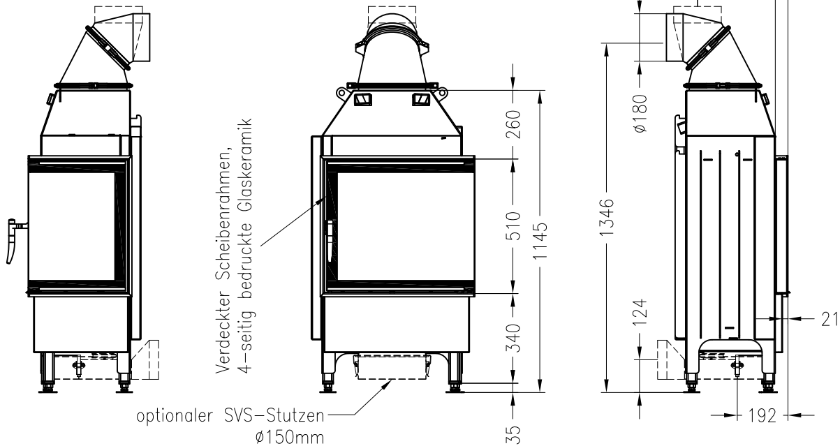
Horizontalschnitt M~1:10
