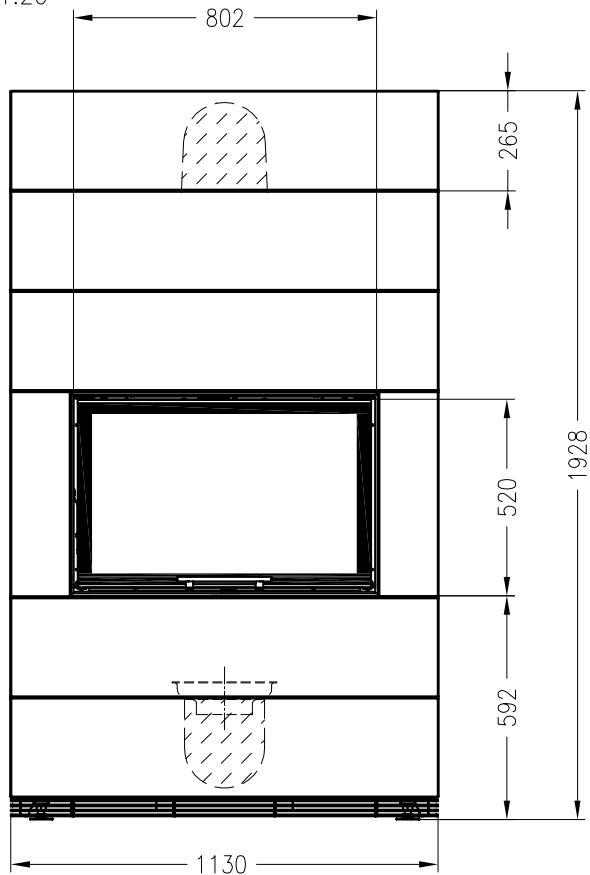
Vorderansicht M~1:20
