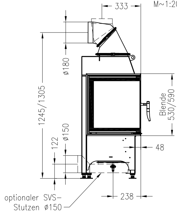
Seitenansicht M~1:20
