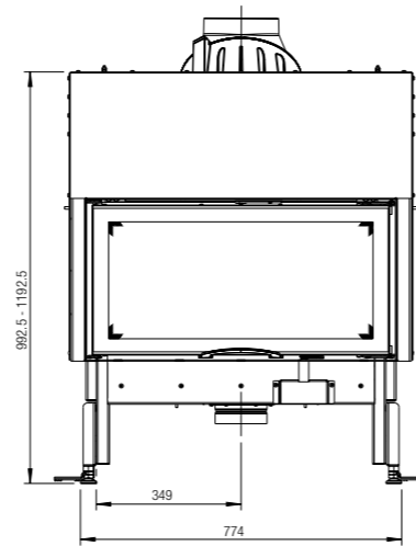
Maßstab 1:20
