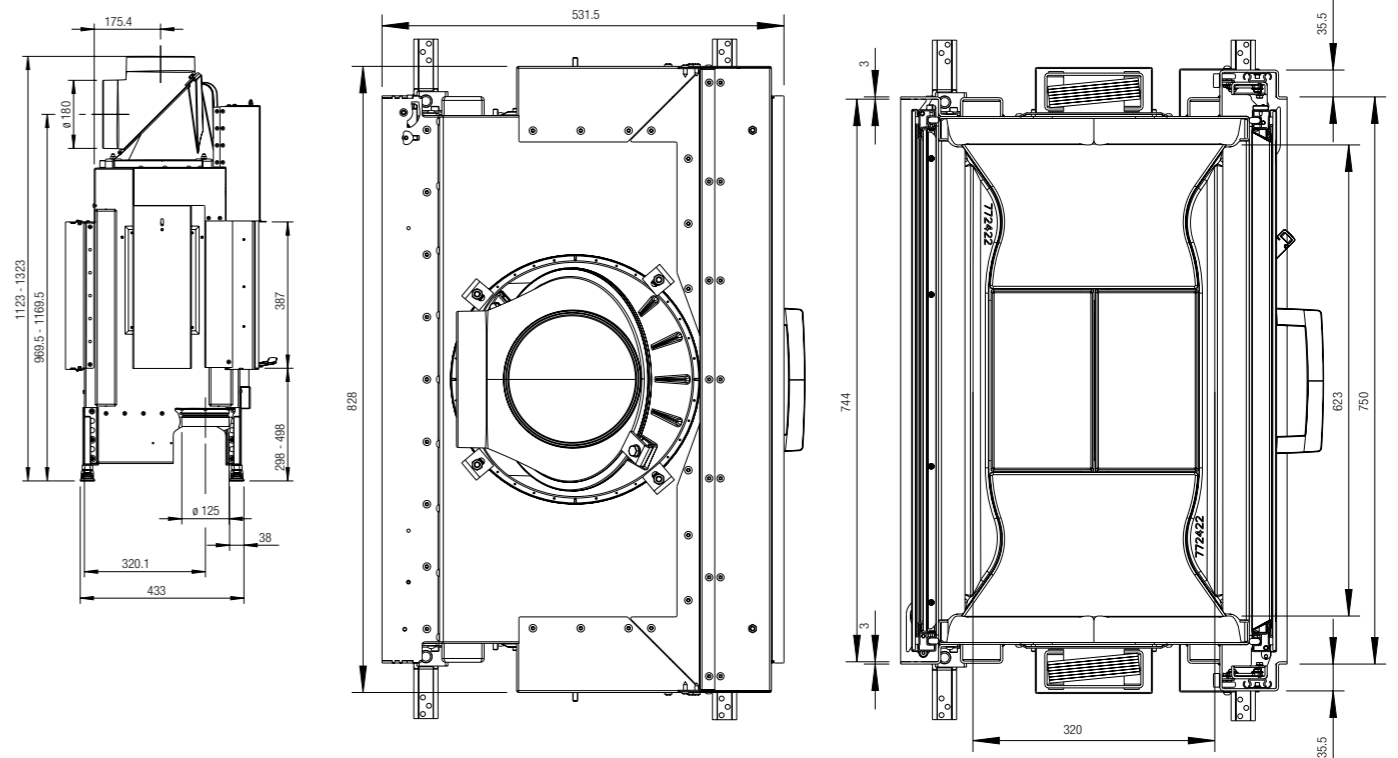
Maßstab 1:10
