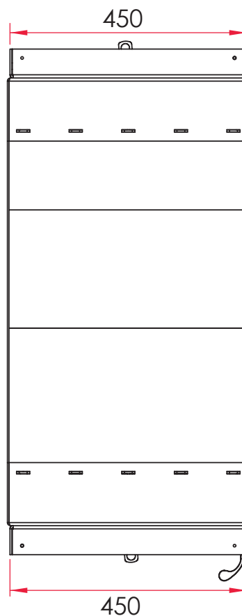
Draufsicht M 1:10
