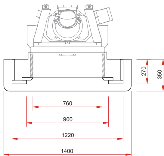
Draufsicht M 1:25
