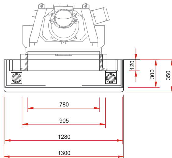
Draufsicht M 1:25
