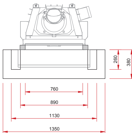
Draufsicht M 1:25
