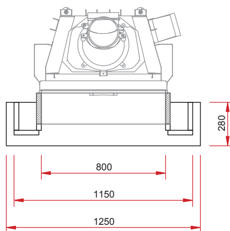
Draufsicht M 1:25
