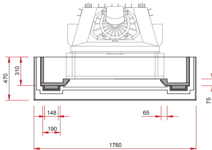
Draufsicht M 1:25
