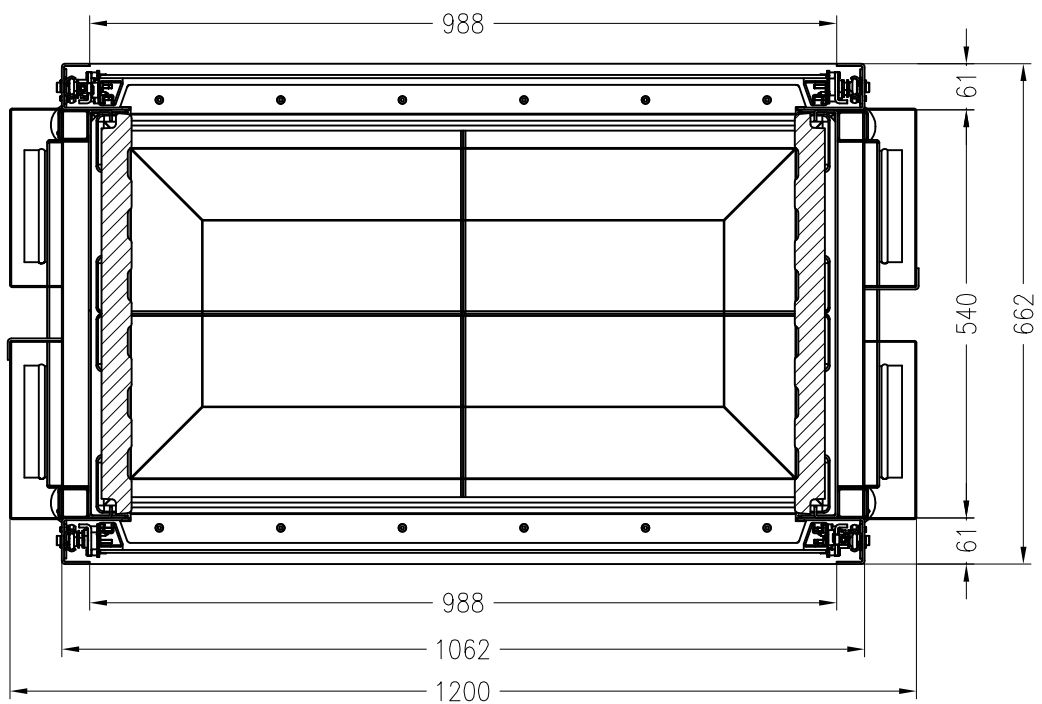
Horizontalschnitt M~1:10
